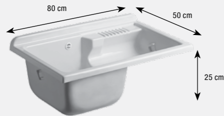
PROFONDITÀ VASCA cm 25 Profondeur vasque cm 25 Tank depth cm 25
